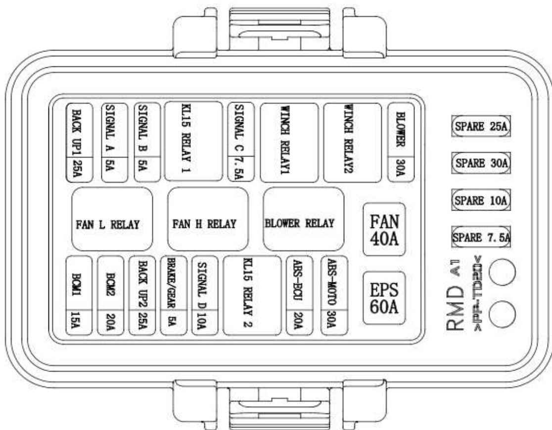
Pojistková skříňka 1 pokud je ve výbavě ABS
