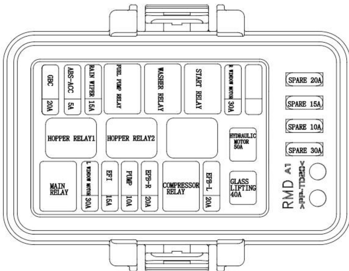
Pojistková skříňka 2 pokud je ve výbavě ABS
