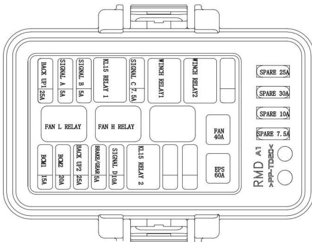
Pojistková skříňka 1 pokud bez ABS
