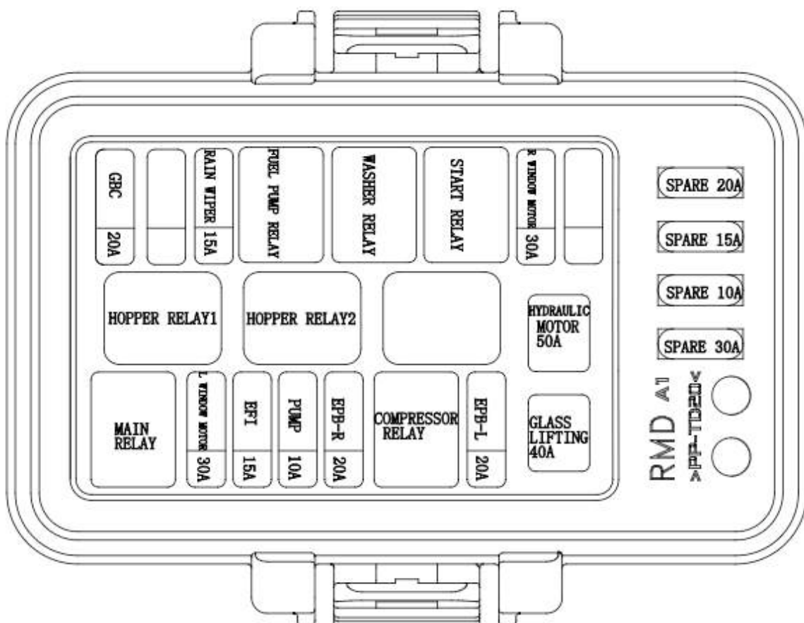
Pojistková skříňka 2 bez ABS
