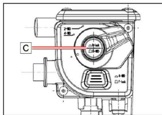
Vozidlá so zadným diferenciálom (EU5)
